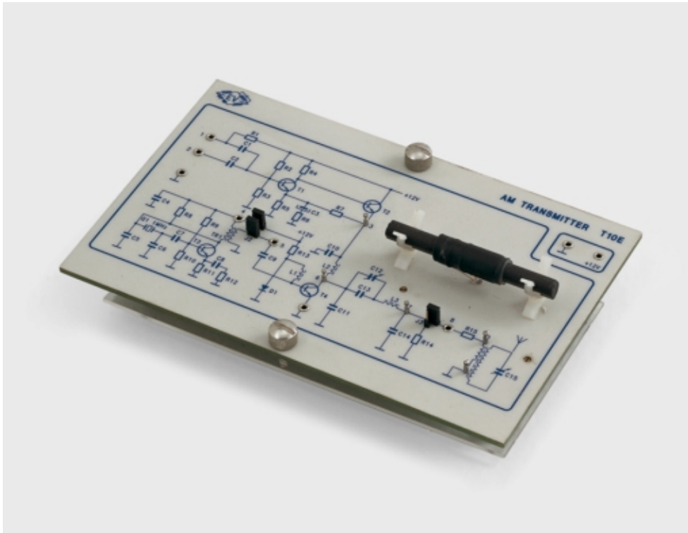
AM TRANSMITTER mod. T10E/EV
